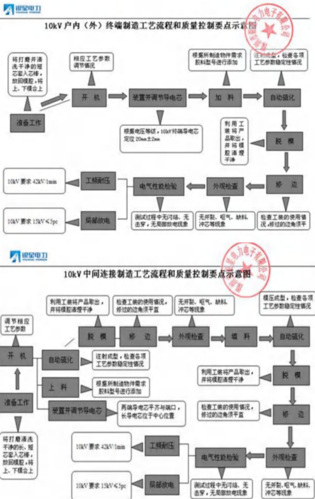
图2：工艺流程
