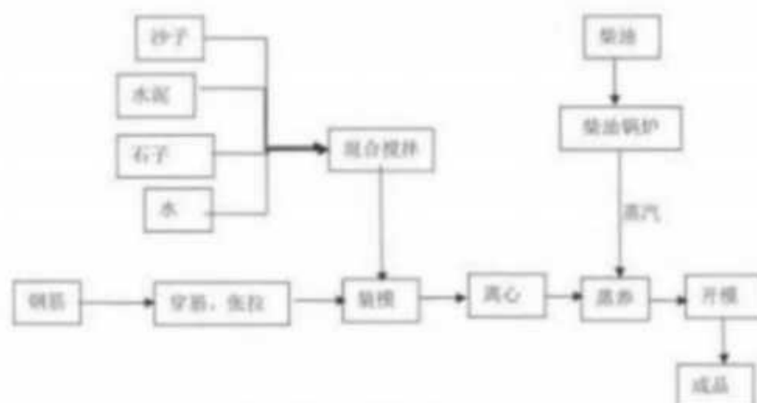
图 1 生产工艺流程图
