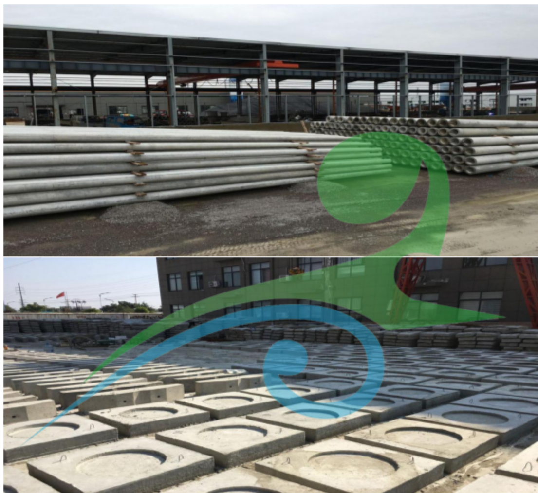
图 2-2 产品概貌
