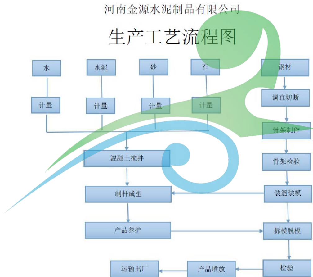
图2-3 产品生产工艺流程
