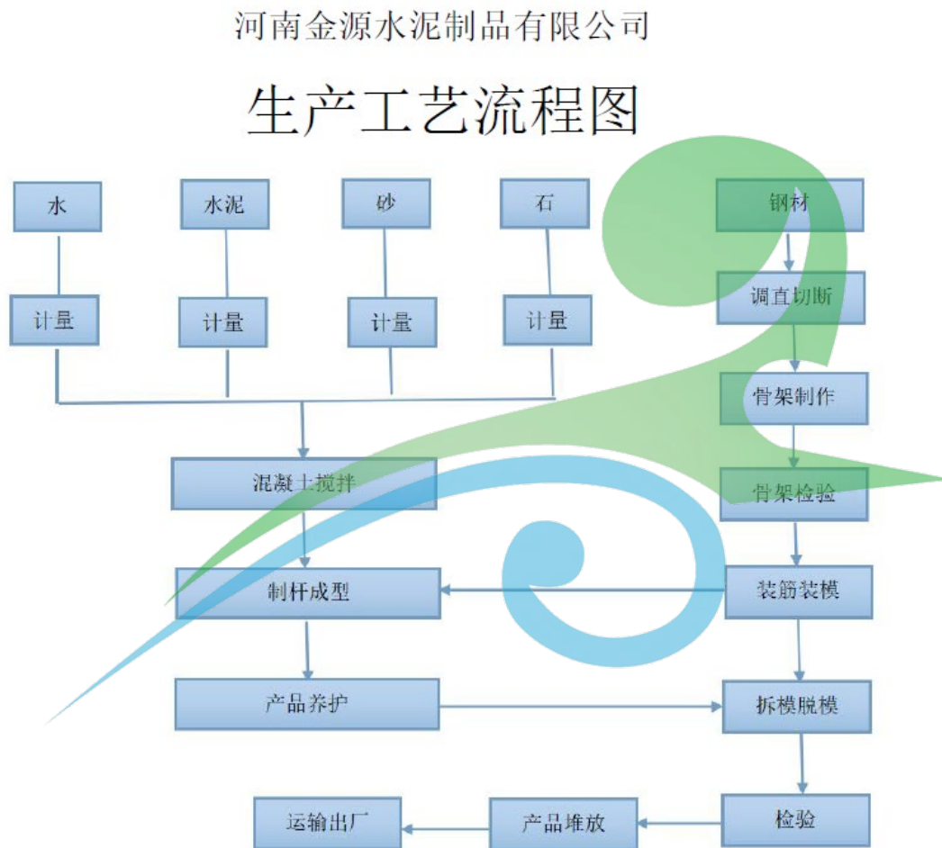
图 2-3 产品生产工艺流程
