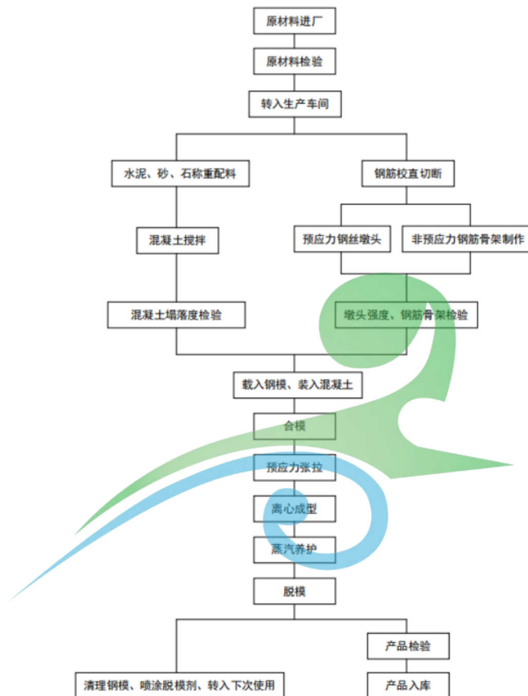
工艺流程图
